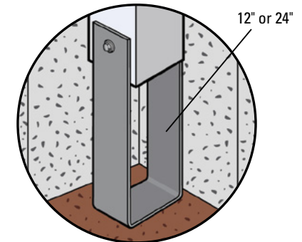
OPTIONAL COLUMN EXTENDER*
